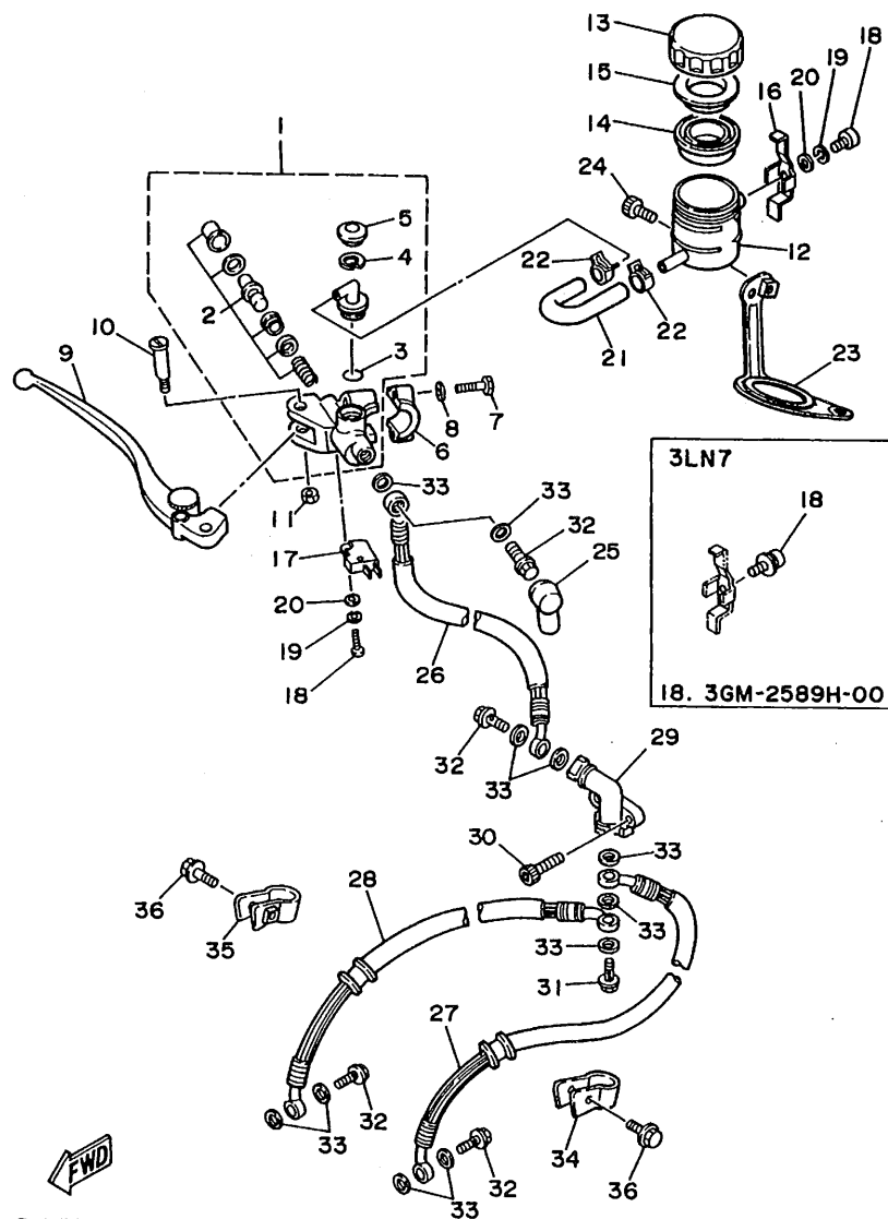
FIG. 35 フロントマスシリンダ 2 (3LN3,5,6,7)
