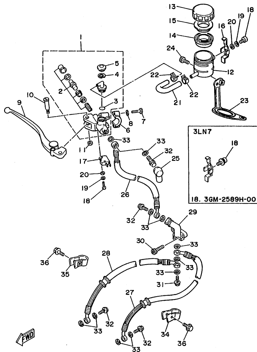
FIG. 35 フロントマスタシリンダ 2 (3LN3,5,6,7)
