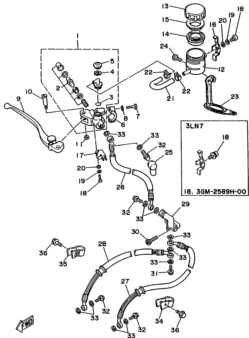
FIG. 35 フロントマスダシリンダ 2 (3LN3,5,6,7)
